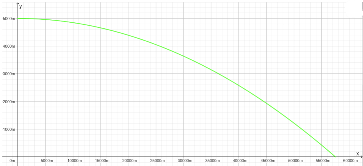
Strecke-Höhe-Diagramm bei einer Notlandung eines Flugzeugs
