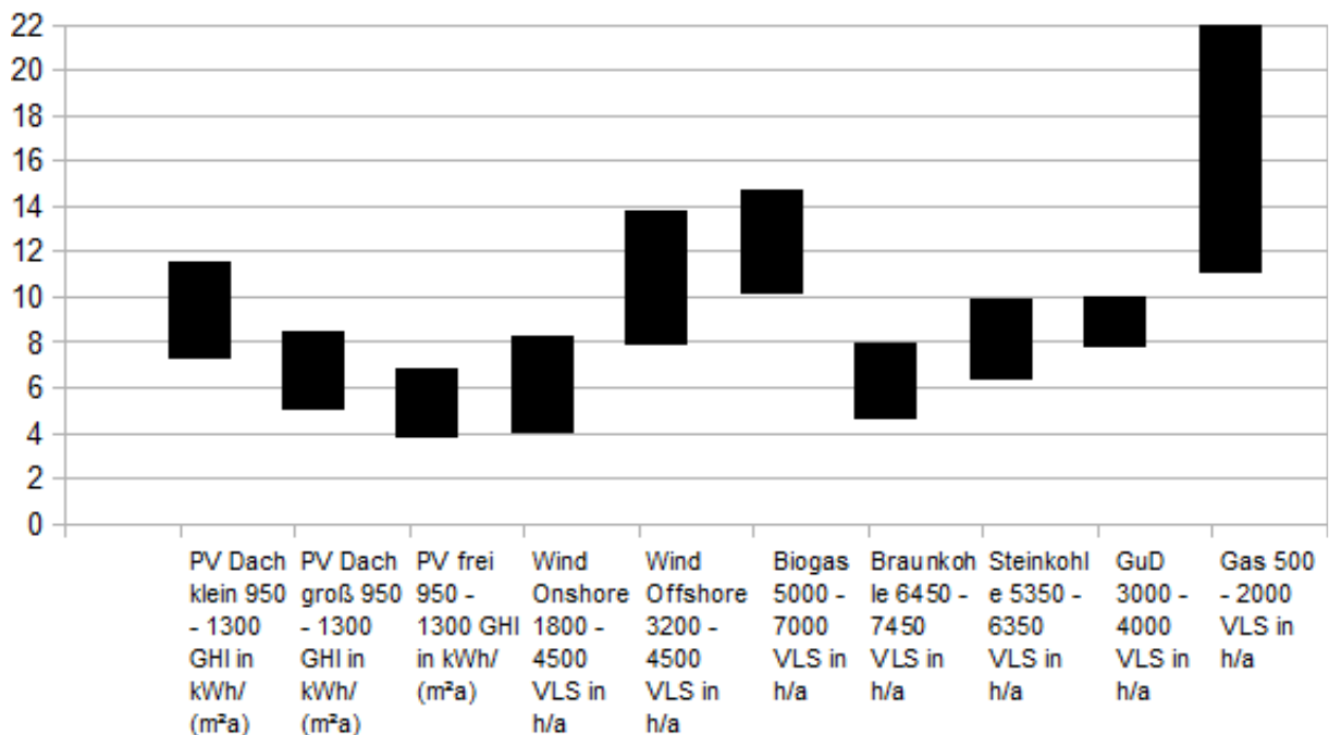
Abb. 2 — Stromgestehungskosten (cent pro kWh) für erneuerbare Energien und konventionelle Kraftwerke an Standorten in Deutschland im Jahr 2018. Der Wert unter der Technologie bezieht sich bei PV auf die solare Einstrahlung (GHI) in kWh/(m 2 a), bei den anderen Technologien gibt sie die Volllaststundenanzahl der Anlage pro Jahr an. Spezifische Anlagekosten sind mit einem minimalen und einem maximalen Wert je Technologie berücksichtigt. Quelle: Fraunhofer ISE
