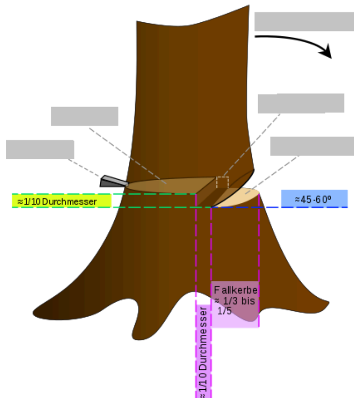
Abb. 1 — Ergänze die fehlende Beschreibung dieses Bildes! Schema des Fallschnitts von Amada44
