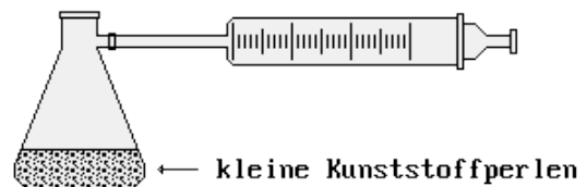
Aufbau zum Ermitteln der molaren Masse
