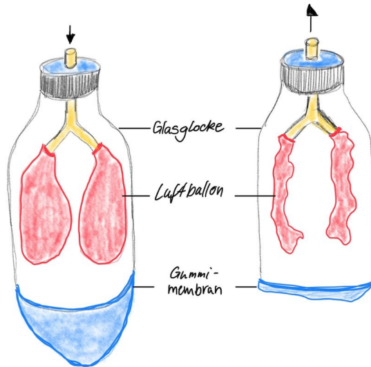
Modell Bauchatmung
