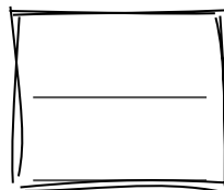
komma- förmig
