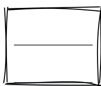
stäbchen- förmig
