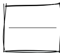
Kokken
