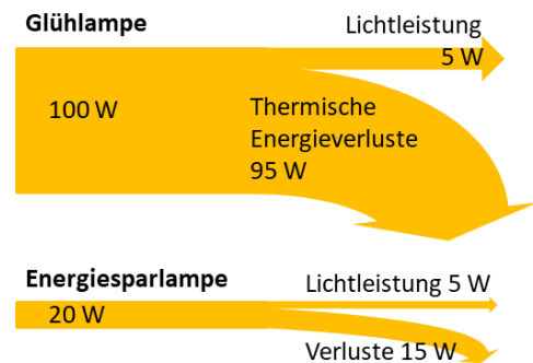
Abb. 1 — Wirkungsgrad einer Glühlampe und einer Energiesparlampe
