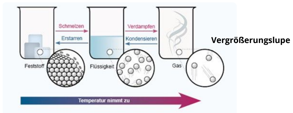
Abbildung 1: Die Teilchenebene
