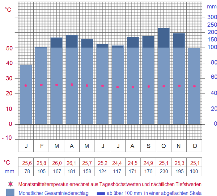
Klimadiagramm Kisangani (Kongo)
