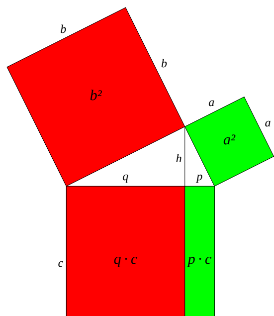
Kathetensatz
