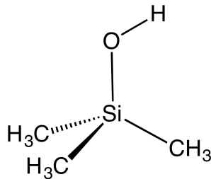
Trimethylsilanol
