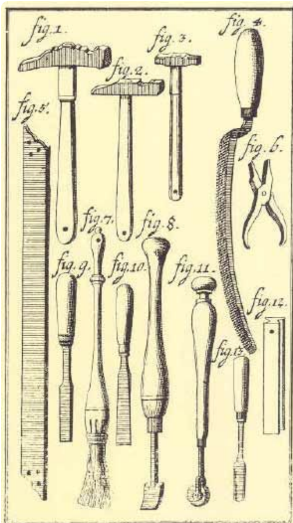
1 Rückenrunde-Hammer – 2 Hammer zum Ableimen – 3 Hämmerlein zum Klausurenanschlagen – 4 Goldschnittraspel – 5 Eisenlineal – 6 Biegezange – 7 Kleisterpinsel – 8 Glättekolben – 9 Stechbeitel – 10 Stemmeisen – 11 Gravierte Rolle für gepunzte Goldschnitte – 12 Einreibehölzchen für Bünde (Vorläufer der Bündezange) – 13 Eckenabstosseisen.
