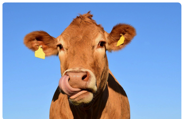
Kuh
