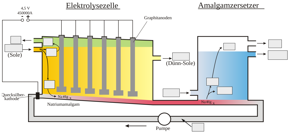
Das nicht mehr gebräuchliche Amalgam-Verfahren
