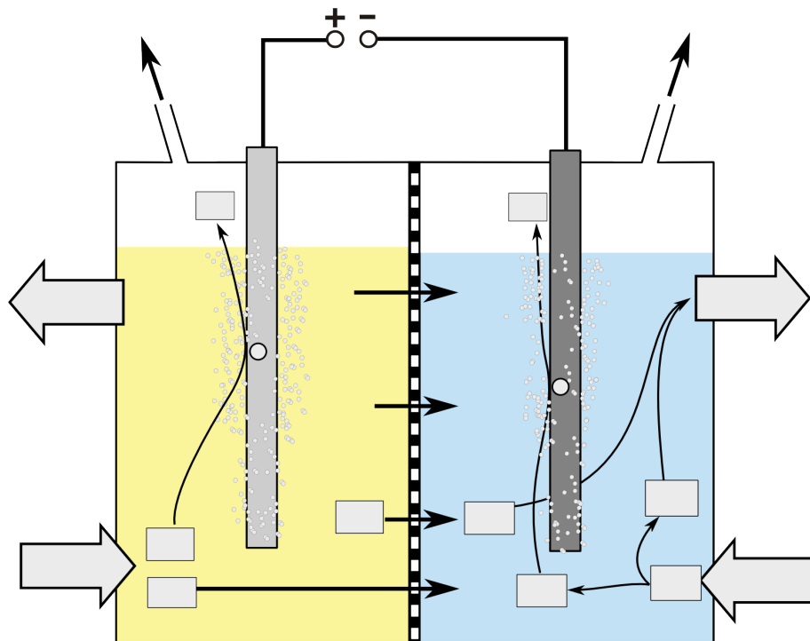
Das modernere Membran-Verfahren
