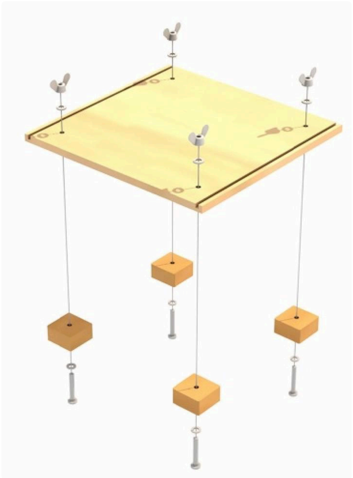
Montage Boden
