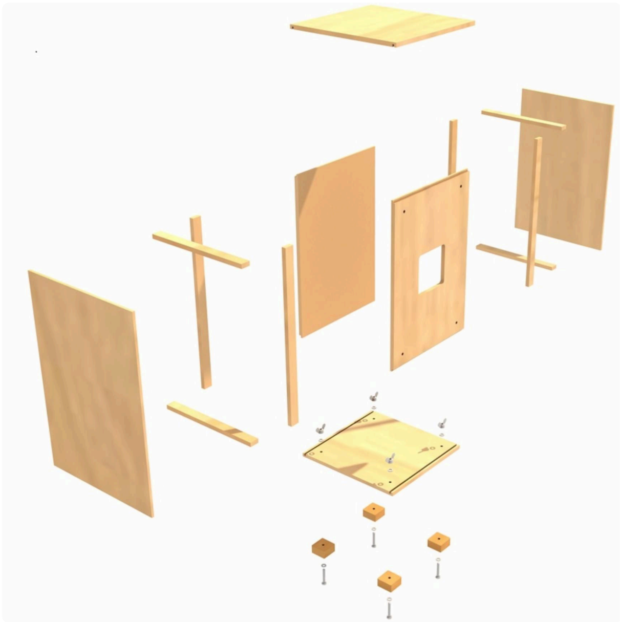
Explosionsbild Cajon
