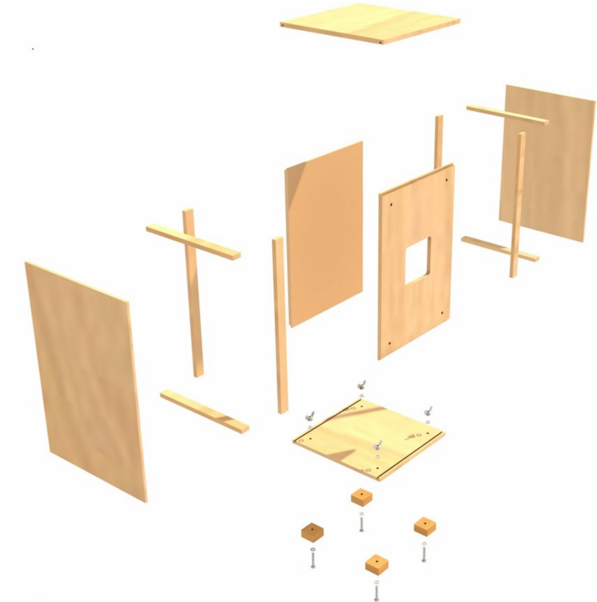
Explosionsbild Cajon
